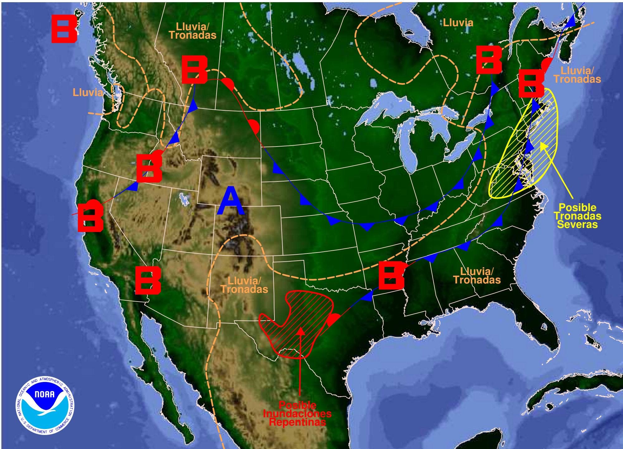
Pronóstico del Tiempo para el Lun 28 de Jun de 2010 emitido 4:30 PM EDT DOC/NOAA/NWS/NCEP/Hydrometeorological Prediction Center Preparado por Hamrick basado en pronósticos del HPC, SPC, y TPC
